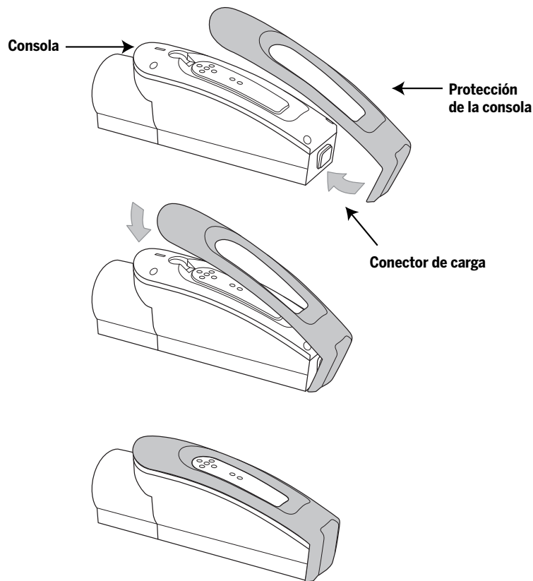
Figura 1. Cómo desmontar o instalar la protección de la consola
