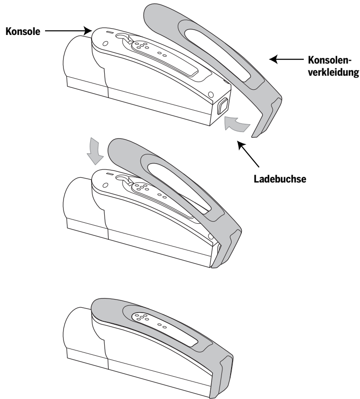
Abbildung 1. Die Konsolenverkleidung abnehmen bzw. aufsetzen
