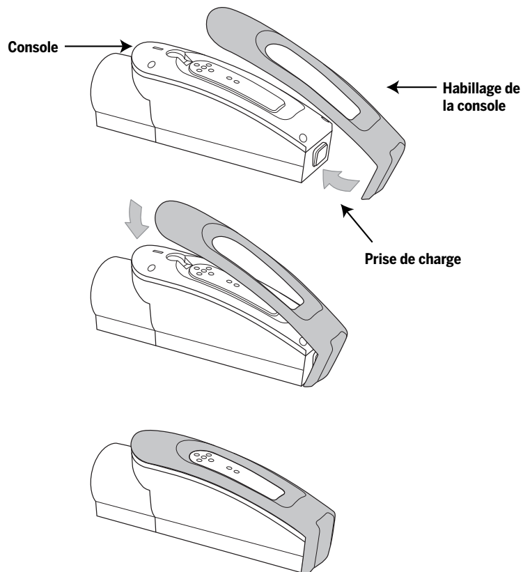
Figure 1. Retrait ou remplacement de l'habillage de la console
