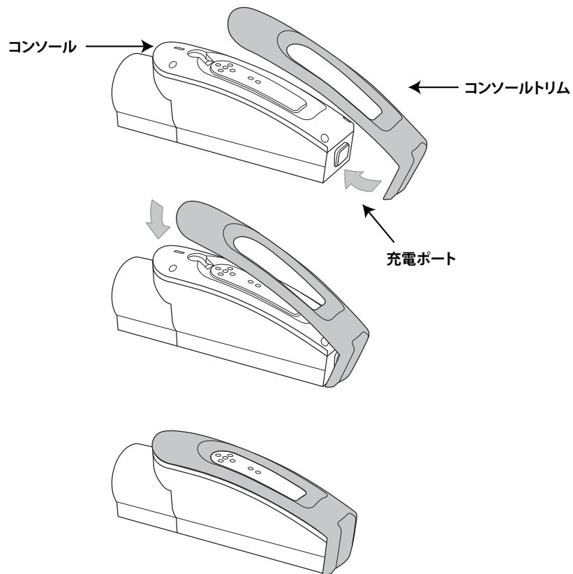
図 1. コンソールトリムの取り外しと取り付け
